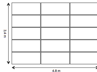
2 montage-varianter med CIS-solcelle-moduler
