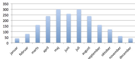
el-produktion i kWh ved 40° hældning stik syd
