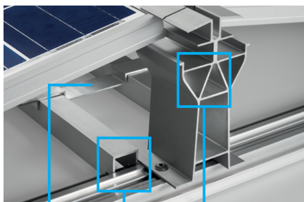
Kombi-klemme Ballastbærer Mellemstøtte
