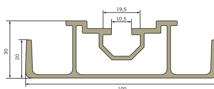
Grundprofil
