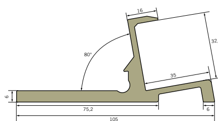
Slutklemme
